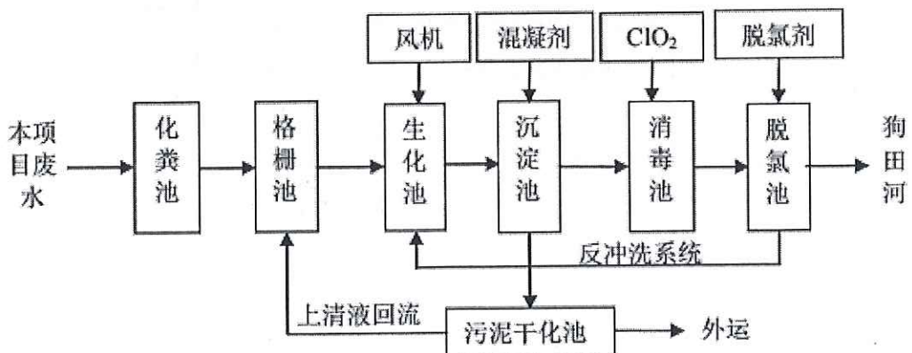
图 2-3 本项目污水处理站工艺流程图
