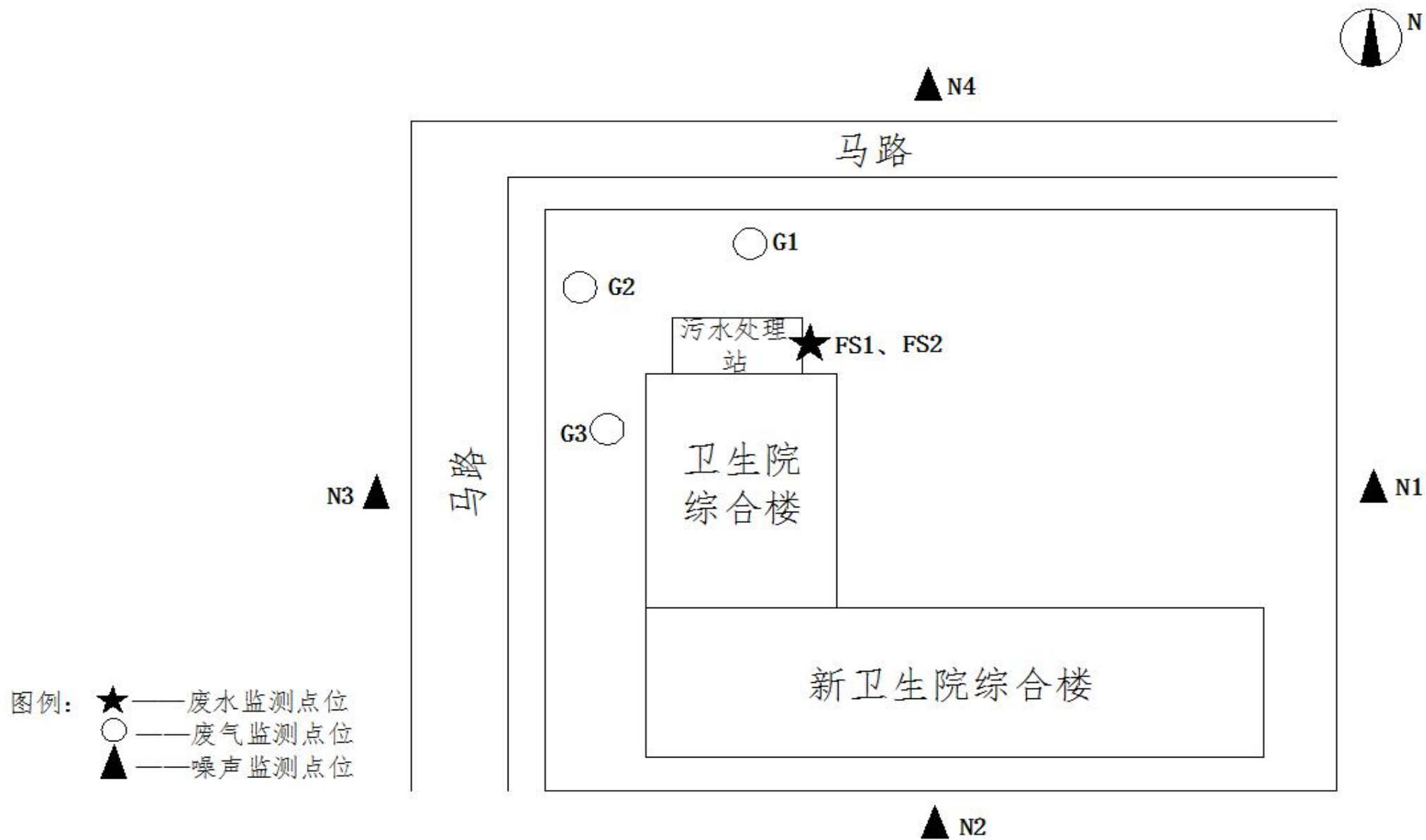
附图 2 平面布置图
