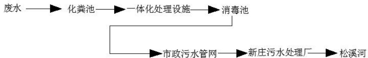
图 3 污水处理流程图
